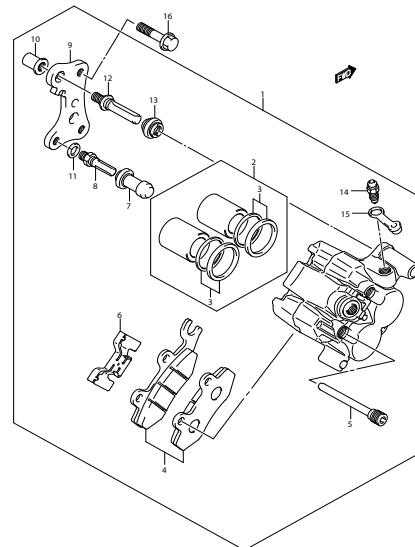
FIG.42A
