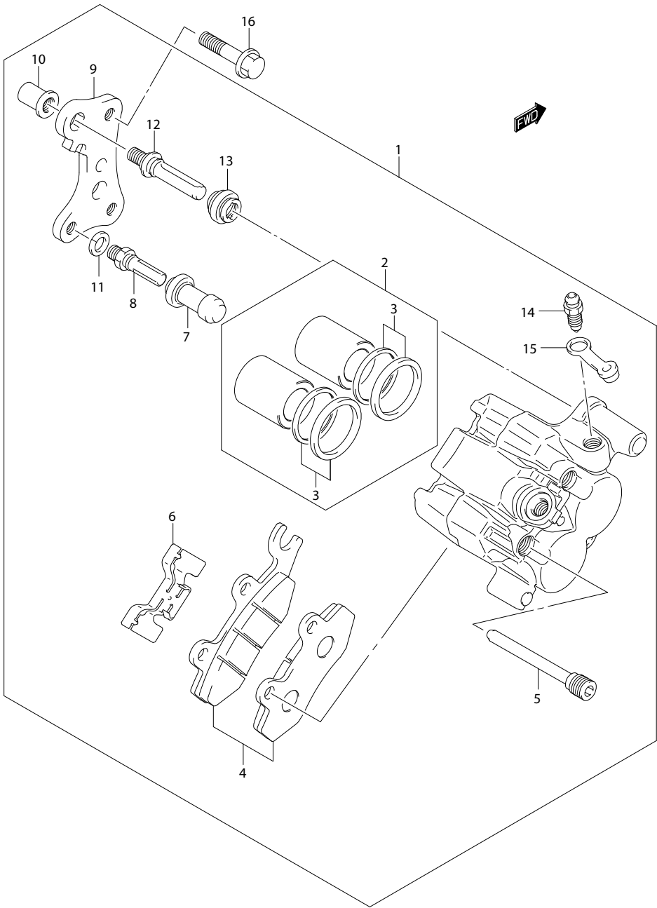
FIG.42A
